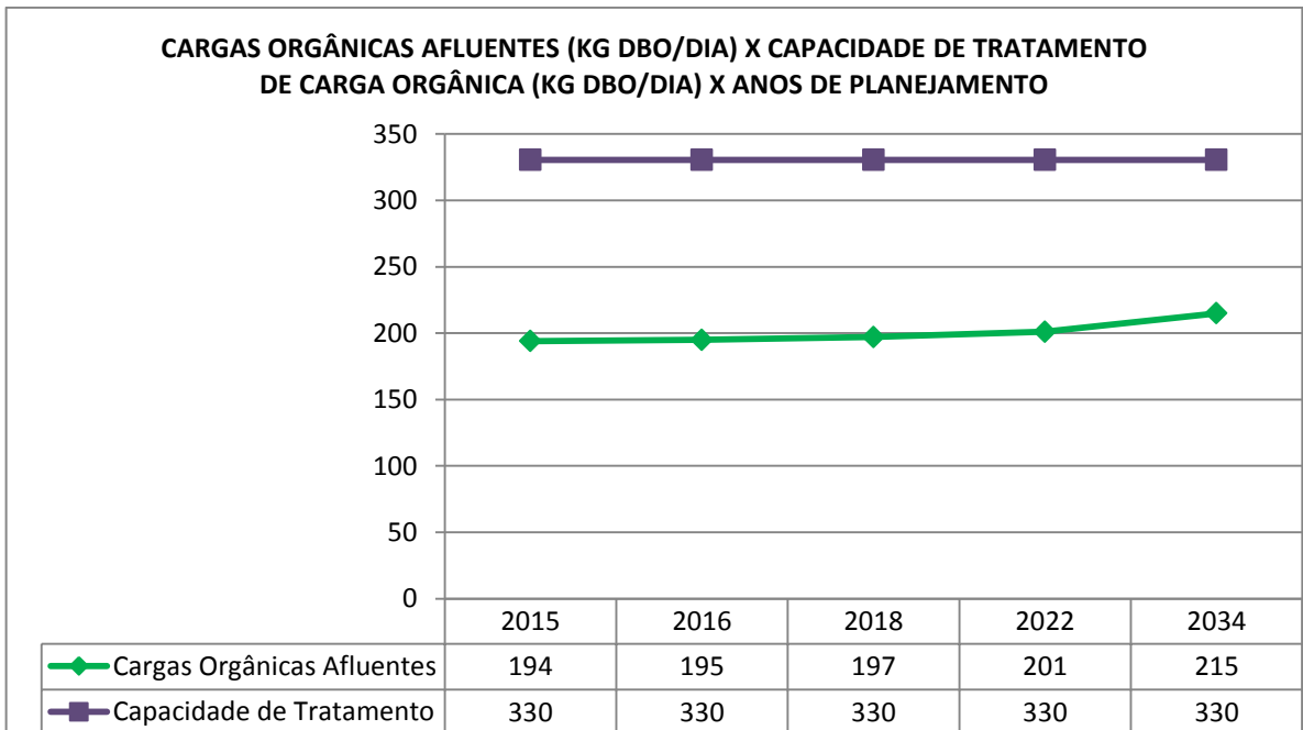
Gráfico 3.6 – Cargas Orgânicas Afluentes (Kg DBO/dia) x Capacidade de Tratamento de Carga Orgânica (kg DBO/dia) x Anos de Planejamento
