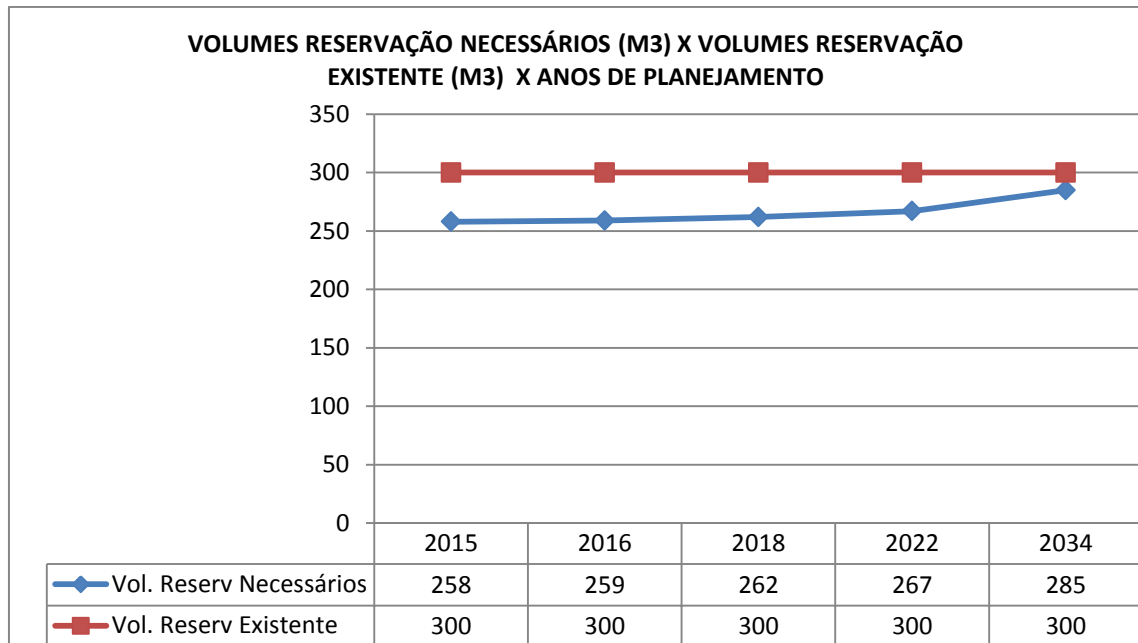
Gráfico 3.3 – Volumes de Reservação Necessários (m 3 ) x Volume de Reservação Existente (m 3 ) x Anos de Planejamento
